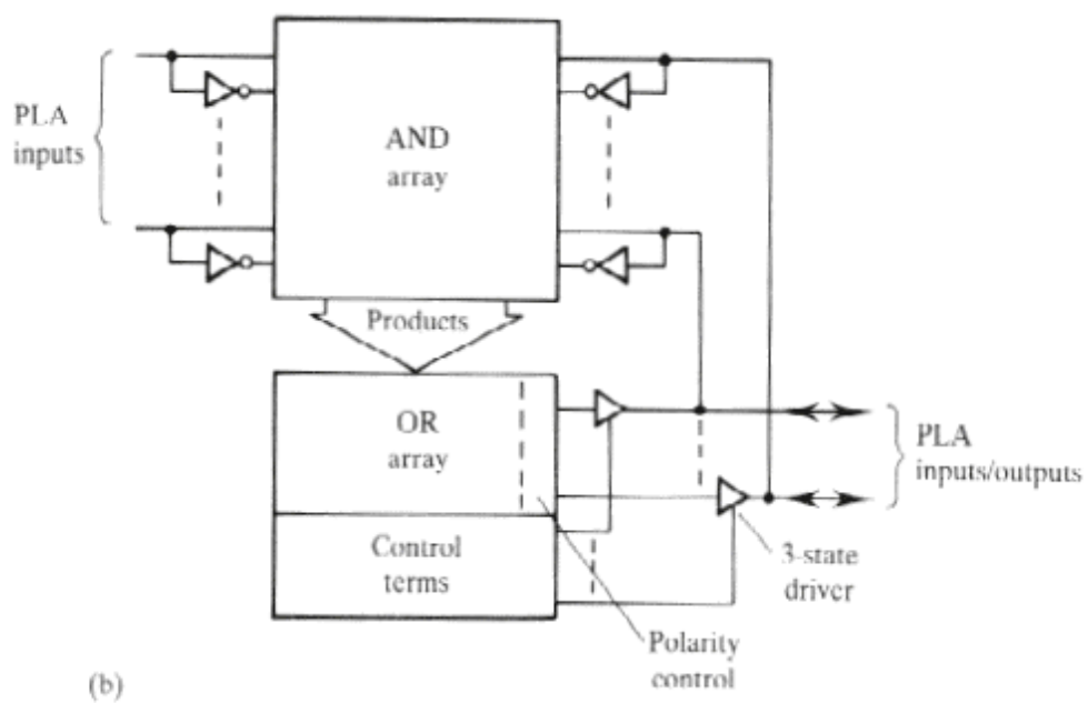
Figura A.1.1. (a) PLA con control de salida. (b) Segunda forma con los terminos de control en OR
