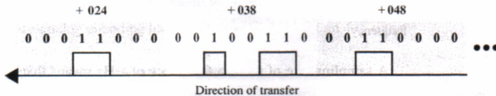
Figura 5 PCM
