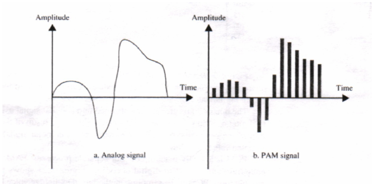
Figura 2 PAM
